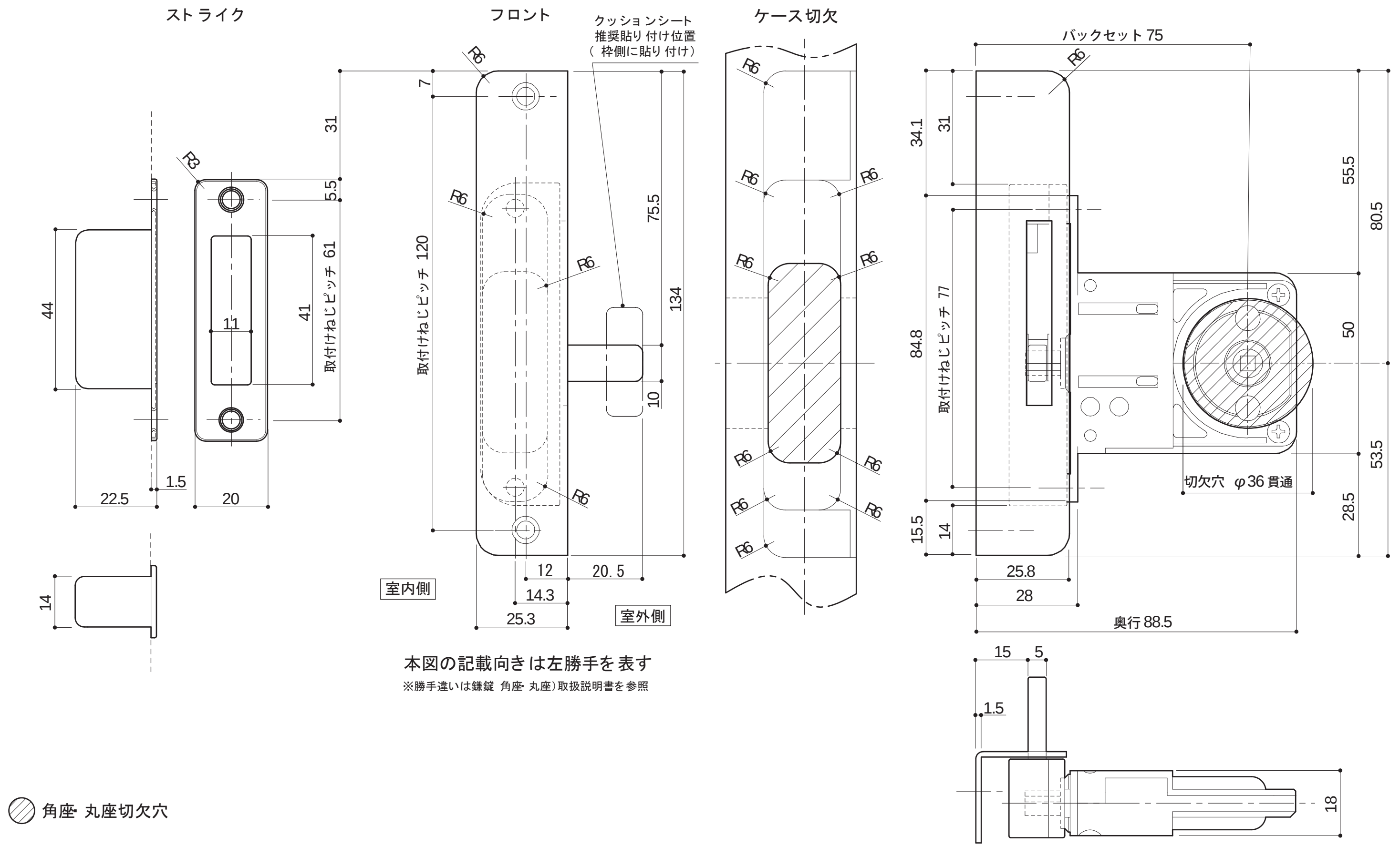
アウトセット引戸錠対応座(KM-17/KM-18/KM-23/KM-24)
